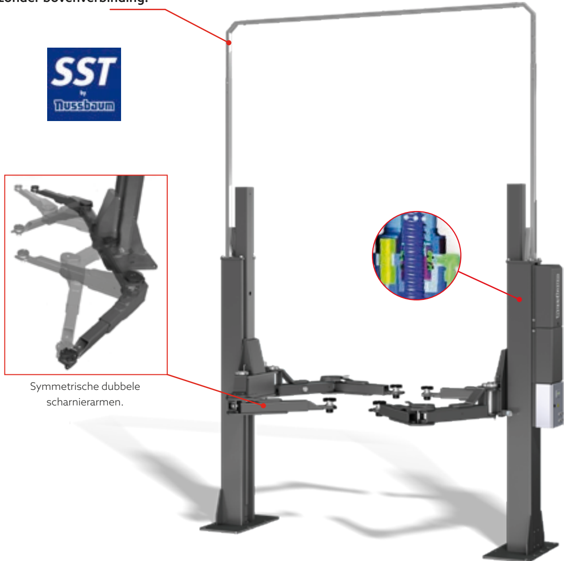
NUSSBAUM POWERLIFT HL 6000 SST DG
